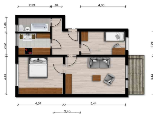
Grundriss
